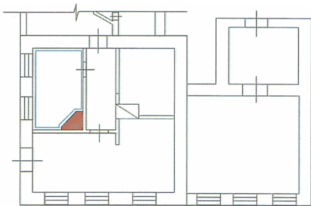
Беренче һәм икенче катларда мич һәм түшәм тартырмасының урнашу урыны
