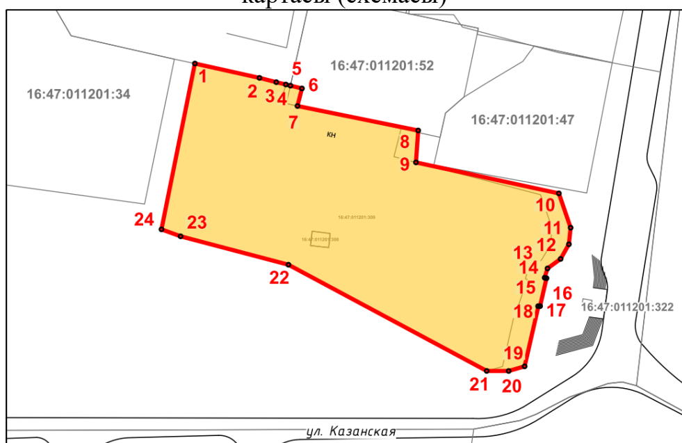
Масштаб 1:1000
