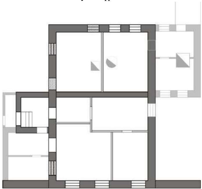
4 рәсем. 1 кат планы
