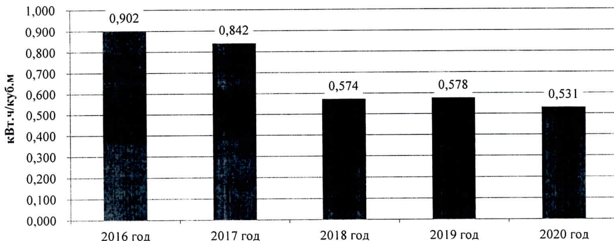
Су бүлү системаларында файдаланыла торган электр энергиясенен чагыштырма чыгымы
