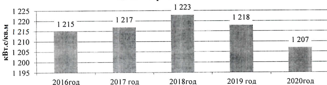
Урамнарны яктырту системаларында электр энергиясенен чагыштырма чыгымы
