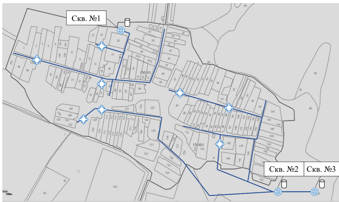
Рисунок 12 Схема водопроводной сети и источников водоснабжения с.Татарский Дюм-Дюм
