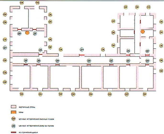
Рис.5. Конструктивная схема
