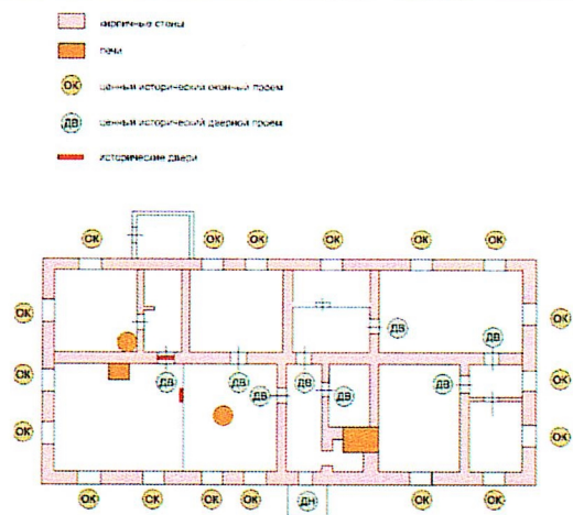
Рис.4. Конструктивная схема
