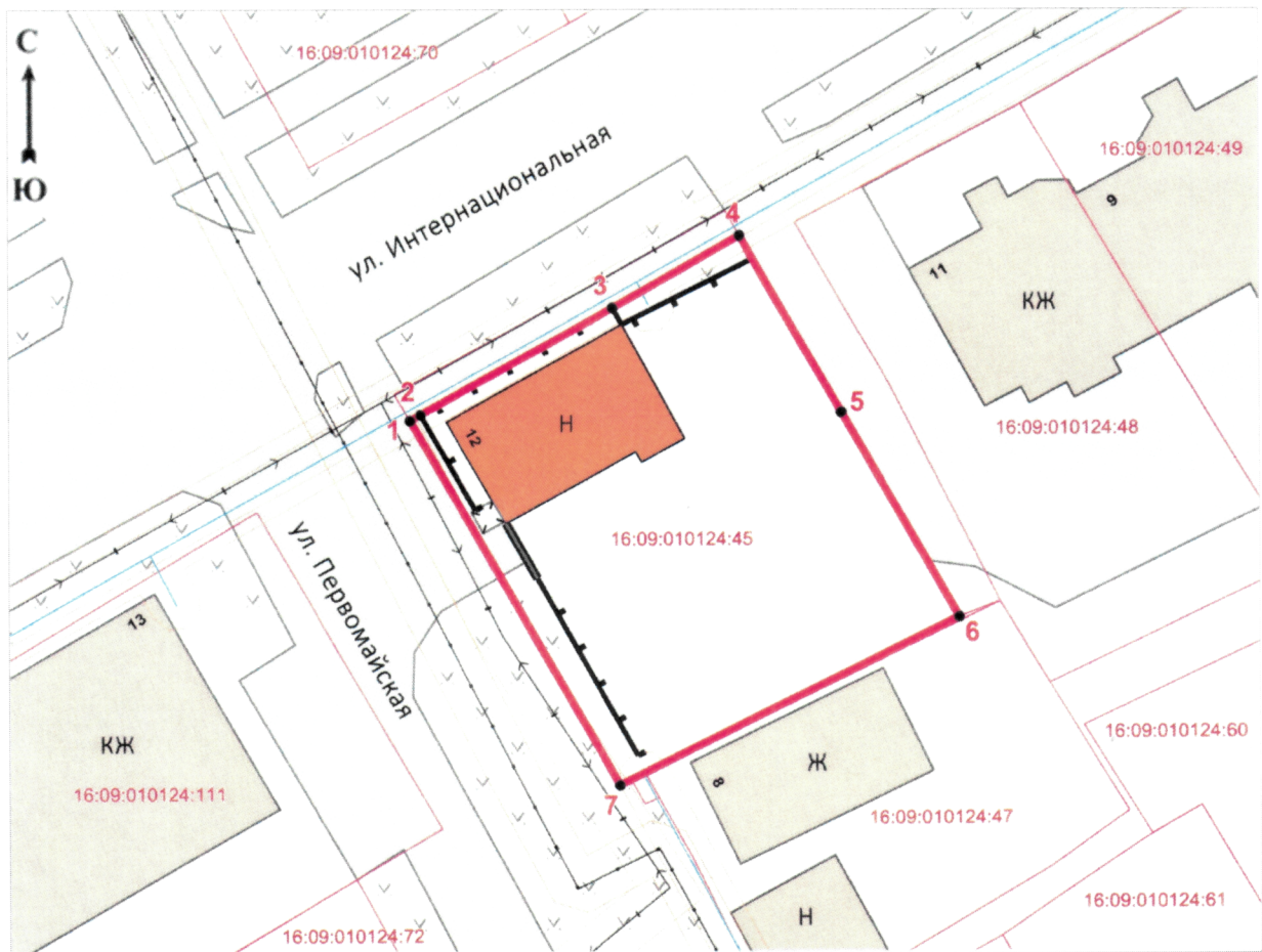
Масштаб 1:600
