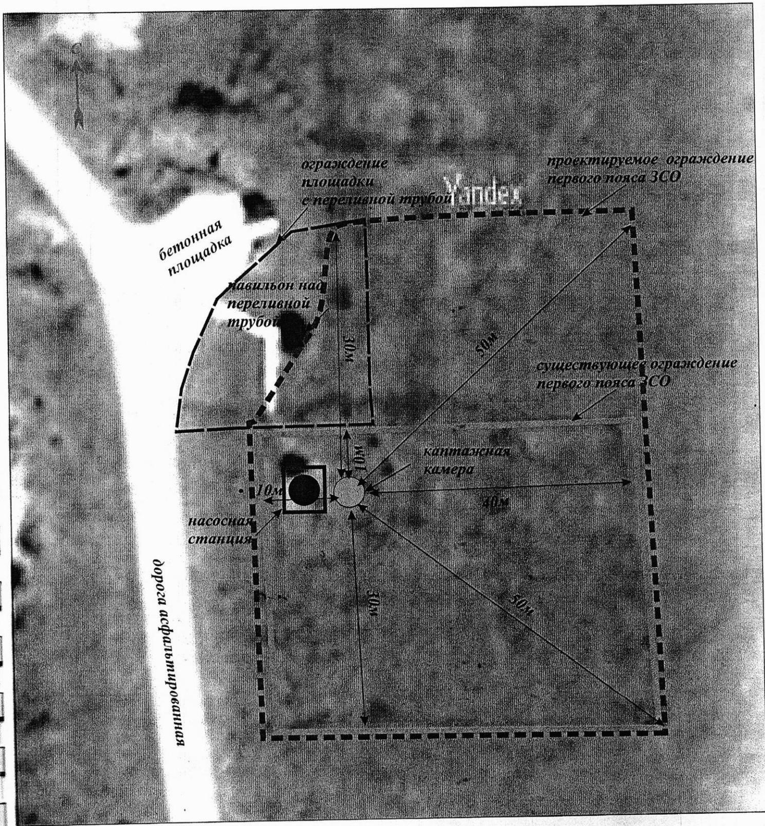
Рис. 4. План-схема границы первого пояса ЗСО родникового водозабора
