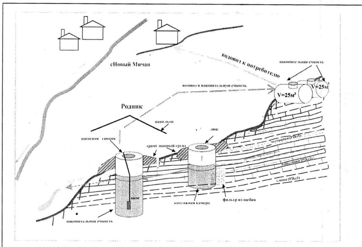
Рис. 12 . Схема каптажа
