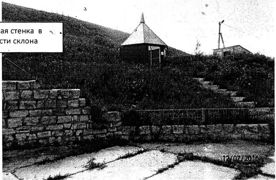
Рис. 9. Родниковый водозабор «Новый Мичан». Павильон над переливной трубой
