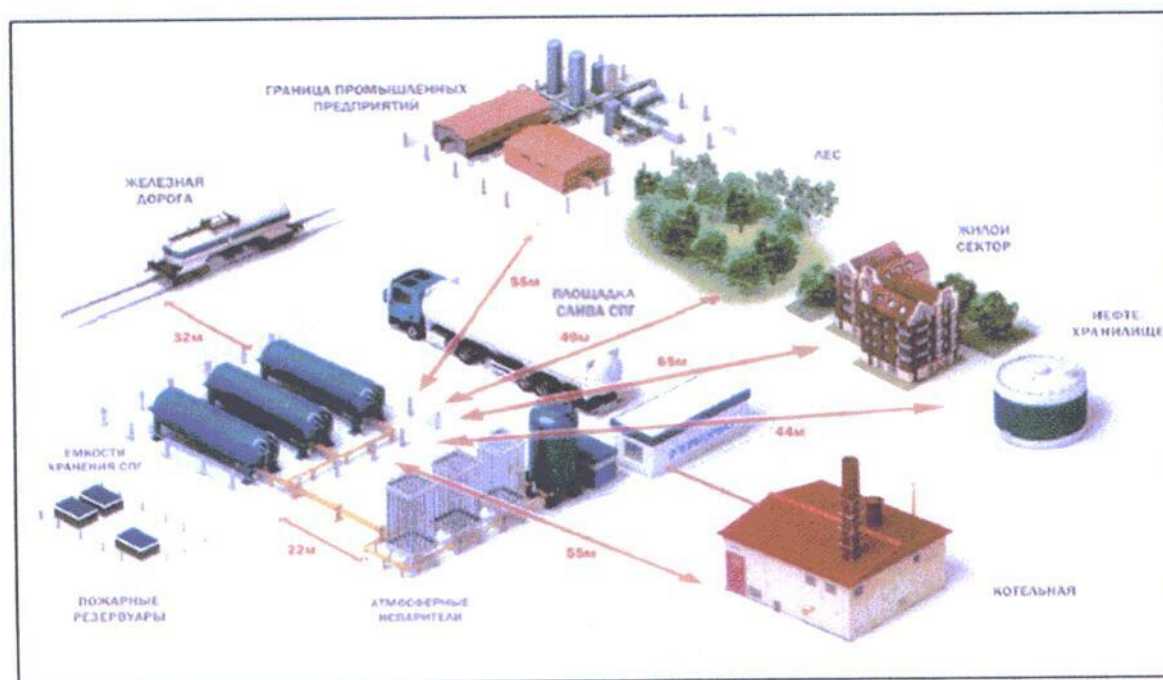
Рис.7. Общий вид производственно-отопительной котельной. Система приема, хранения и регазификации
