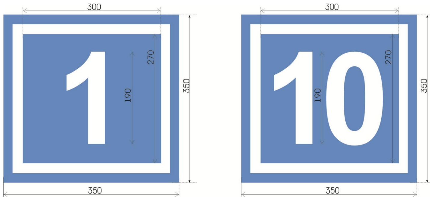
Номерной знак
