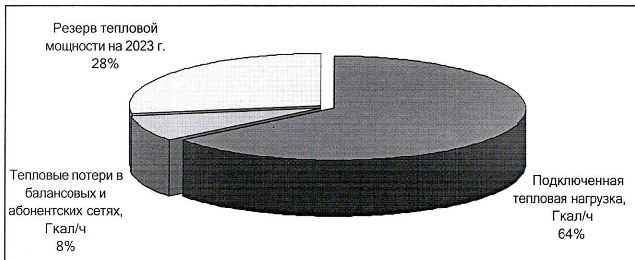
рис. 10. Диаграмма балансов тепловой мощности и подключенных нагрузок на 2 этапе развития схемы теплоснабжения
