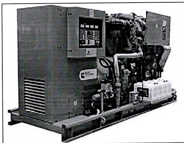
рис. 13 Газопоршневая установка С315 NSC фирмы «Cummins»
