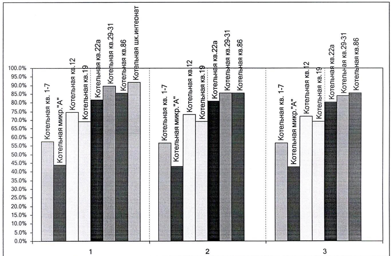
рис. 12 Запас мощности водоподготовительных установок
