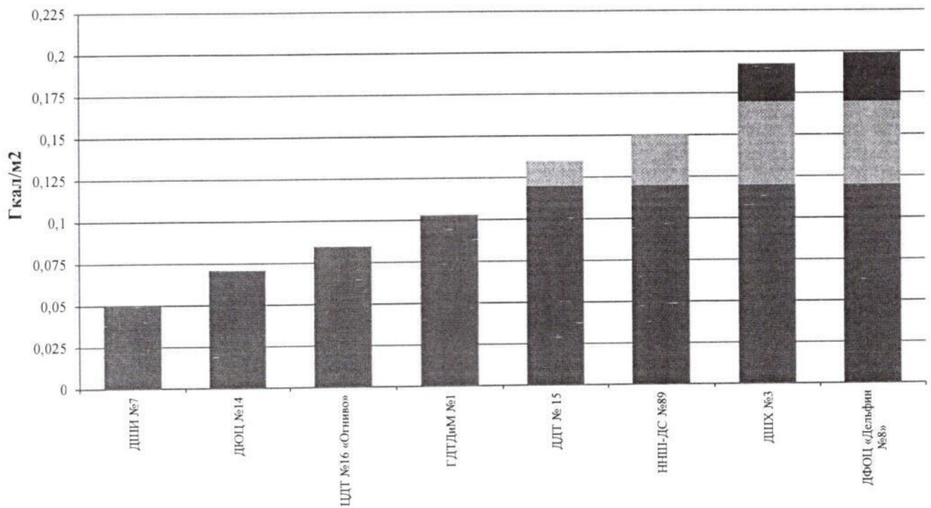
Ранжирование зданий дополнительных образовательных учреждений г.Набережные Челны по удельным расходам тепловой энергии на 1м2 общей площади.
