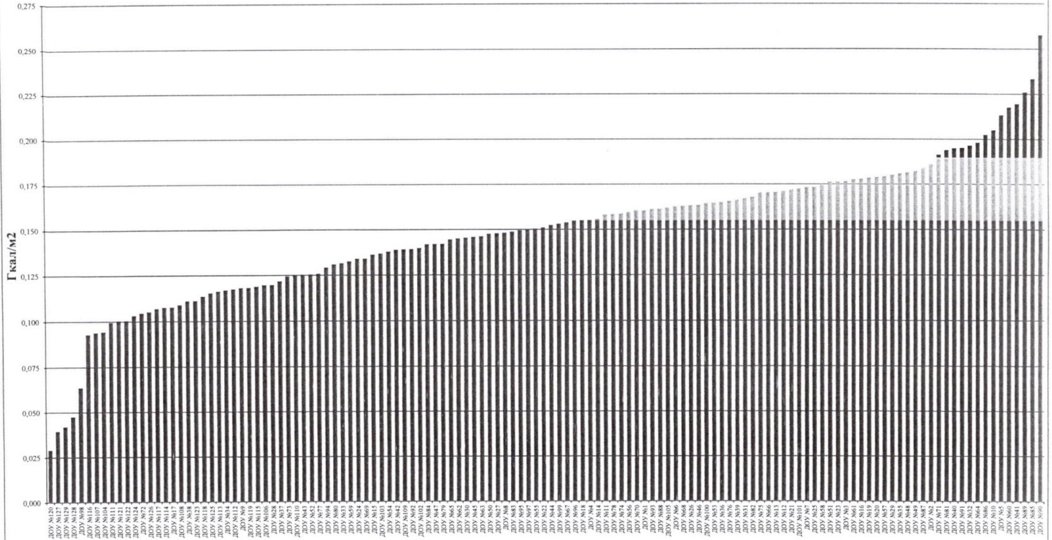
Ранжирование дошкольных образовательных учреждений г.Набережные Челны по удельным расходам тепловой энергии на 1м 2 общей площади.
