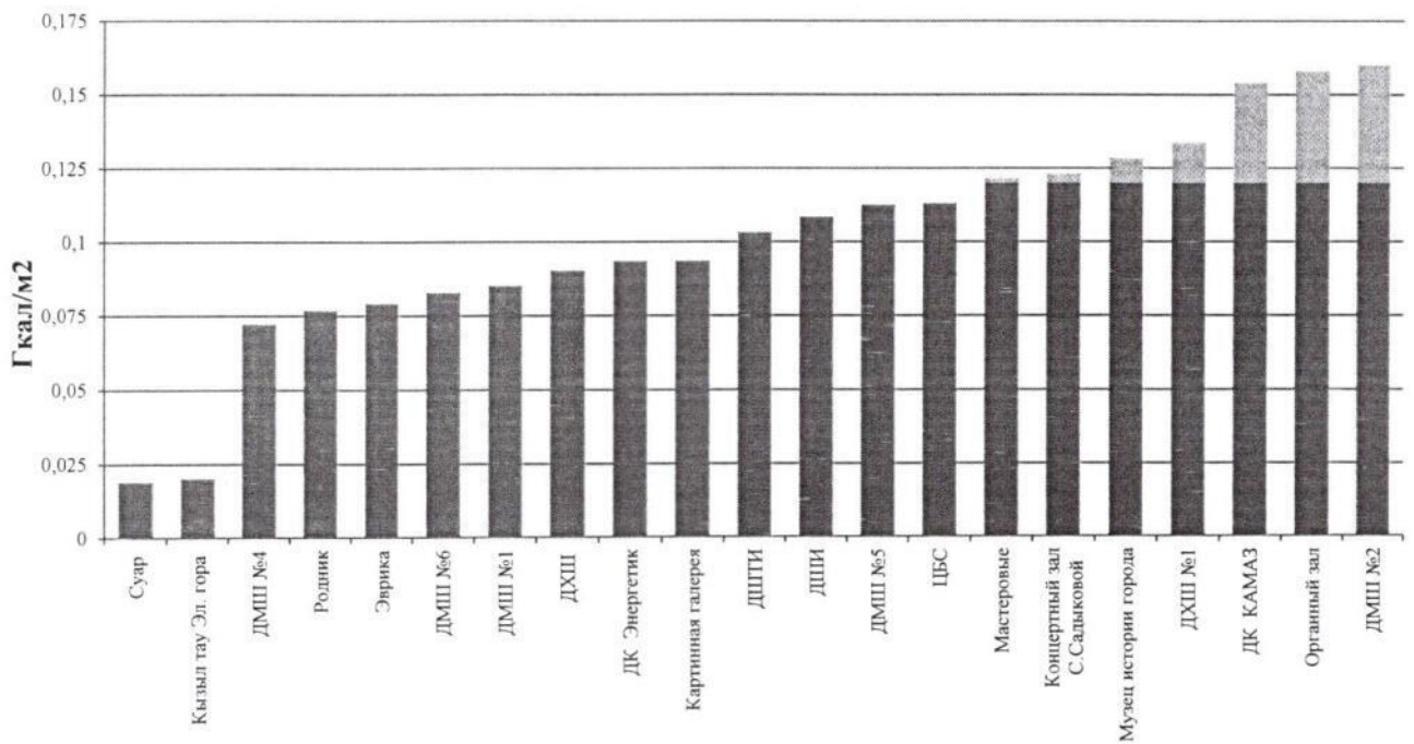
Ранжирование зданий Управления культуры г.Набережные Челны по удельным расходам тепловой энергии на 1м2 общей площади.
