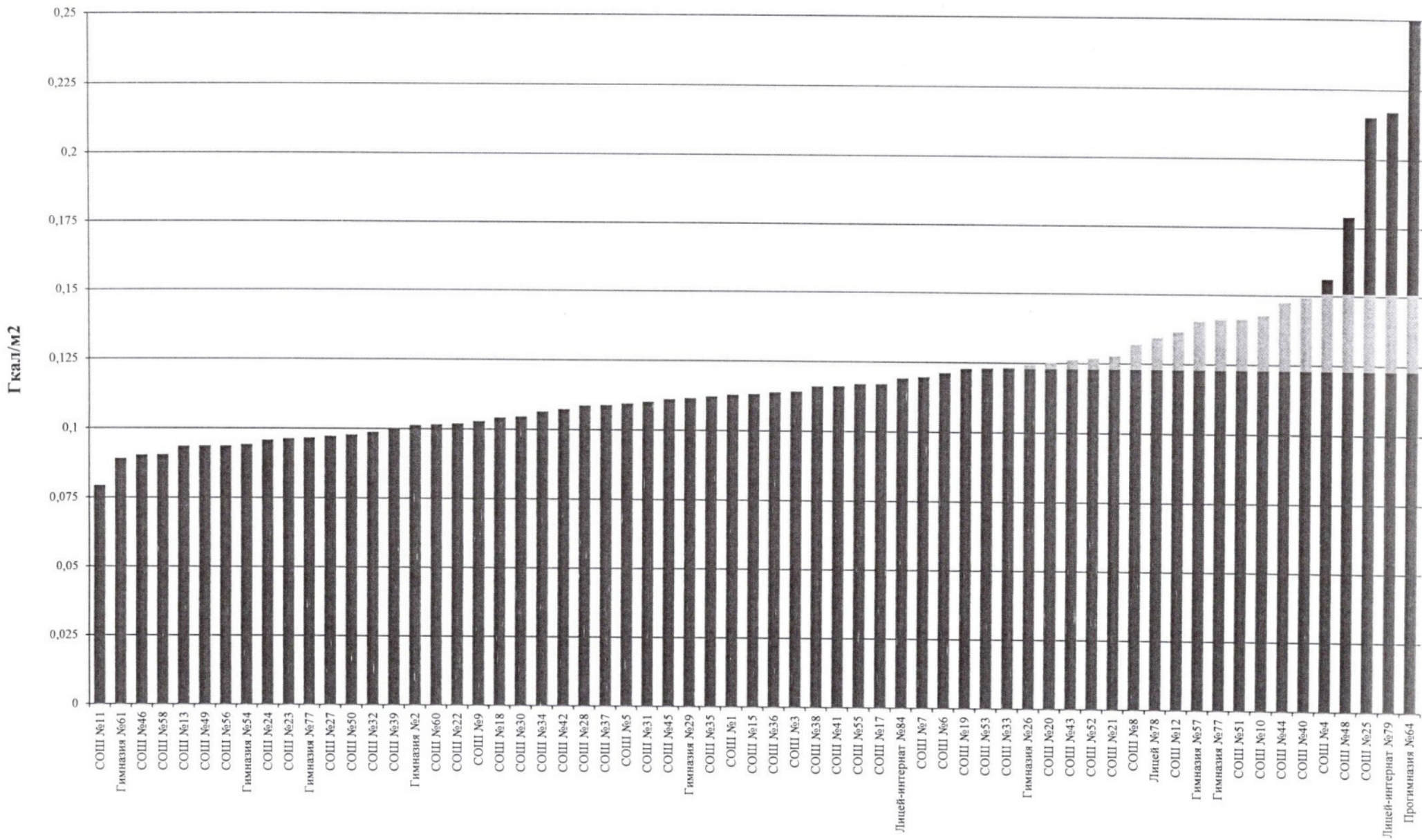
Ранжирование зданий учебных учреждений г.Набережные Челны по удельным расходам тепловой энергии на 1м2 общей площади.
