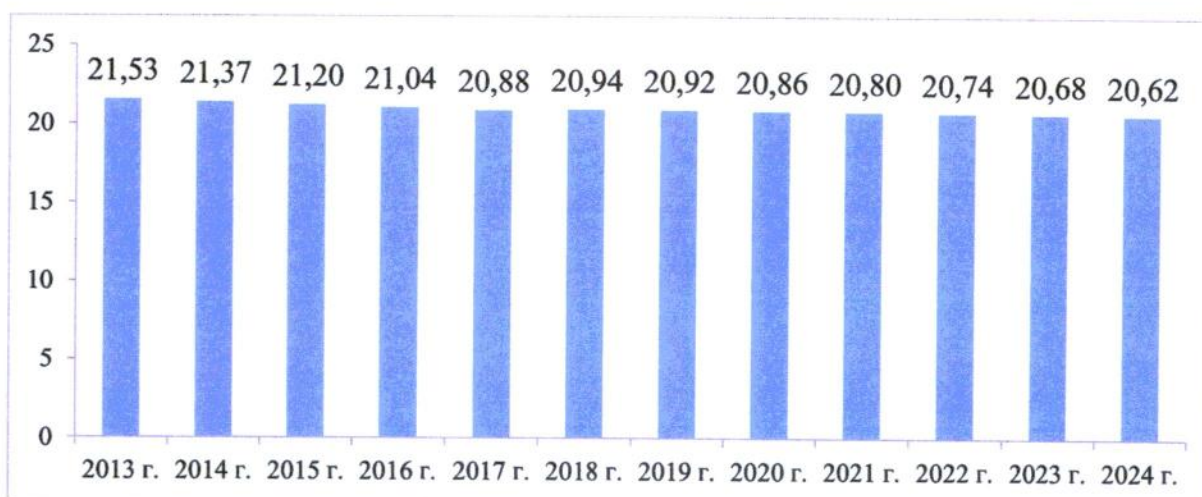
Рис.17. Динамика и прогноз энергоемкости ВРП (т.у.т./млн.рублей);
