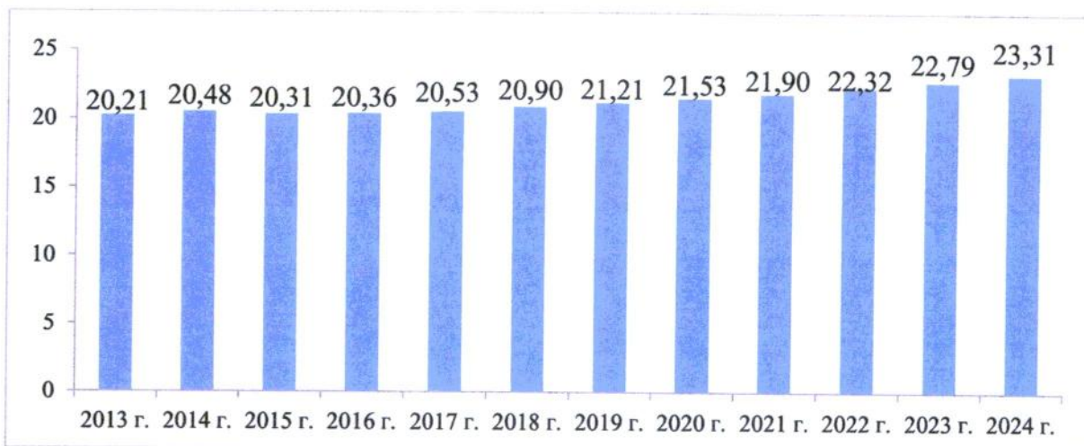
Рис.16. Динамика и прогноз потребления первичных энергоносителей (млн.т.у.т.)
